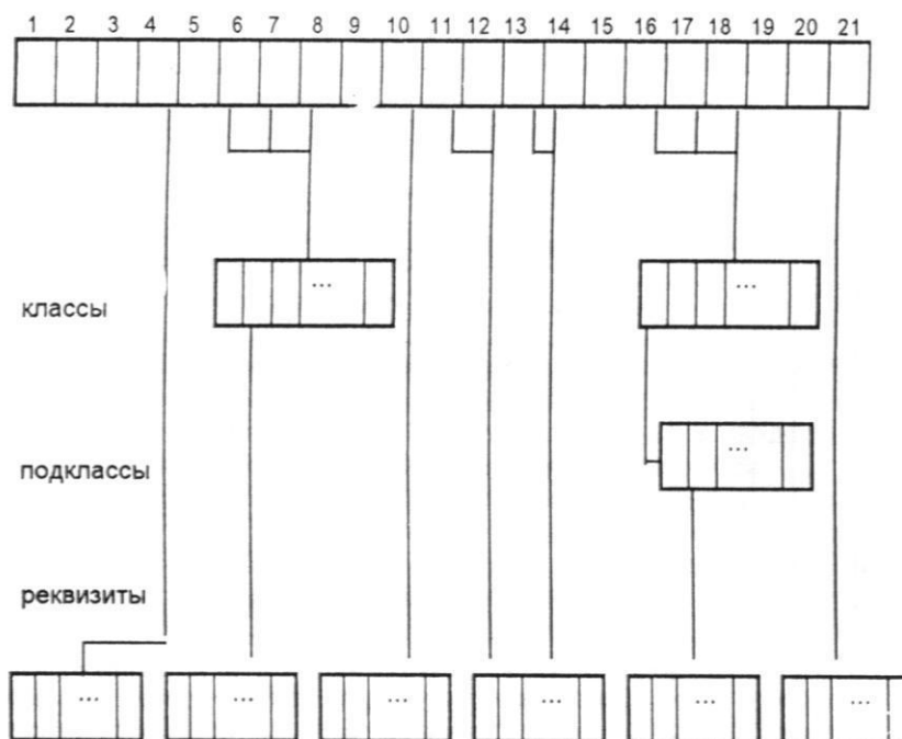
Рис.2. Структура классификатора
