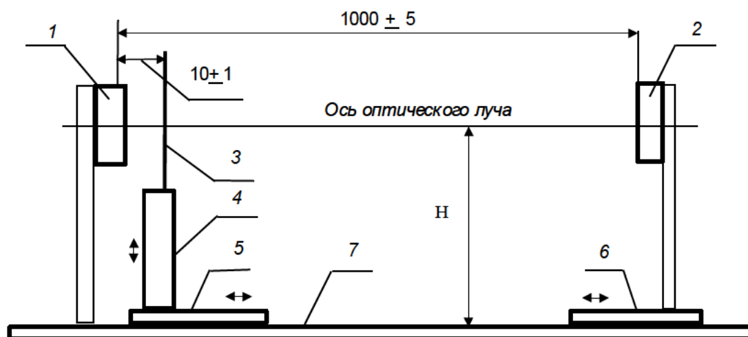
Рис. 1. Схема расположения элементов ИПДЛ и аттенюатора (вариант 1 - передатчик и приемник):
