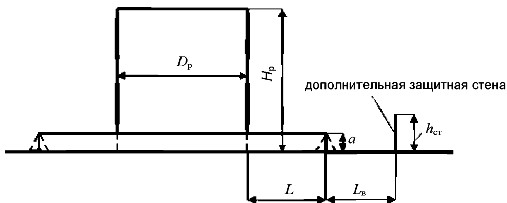
Рисунок Б.1 — Расчетная схема дополнительной защитной стены
