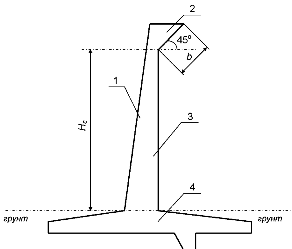
1 — защитная стена; 2 — волноотражающий козырек; 3 — площадка отражения потока; 4 — основание стены
