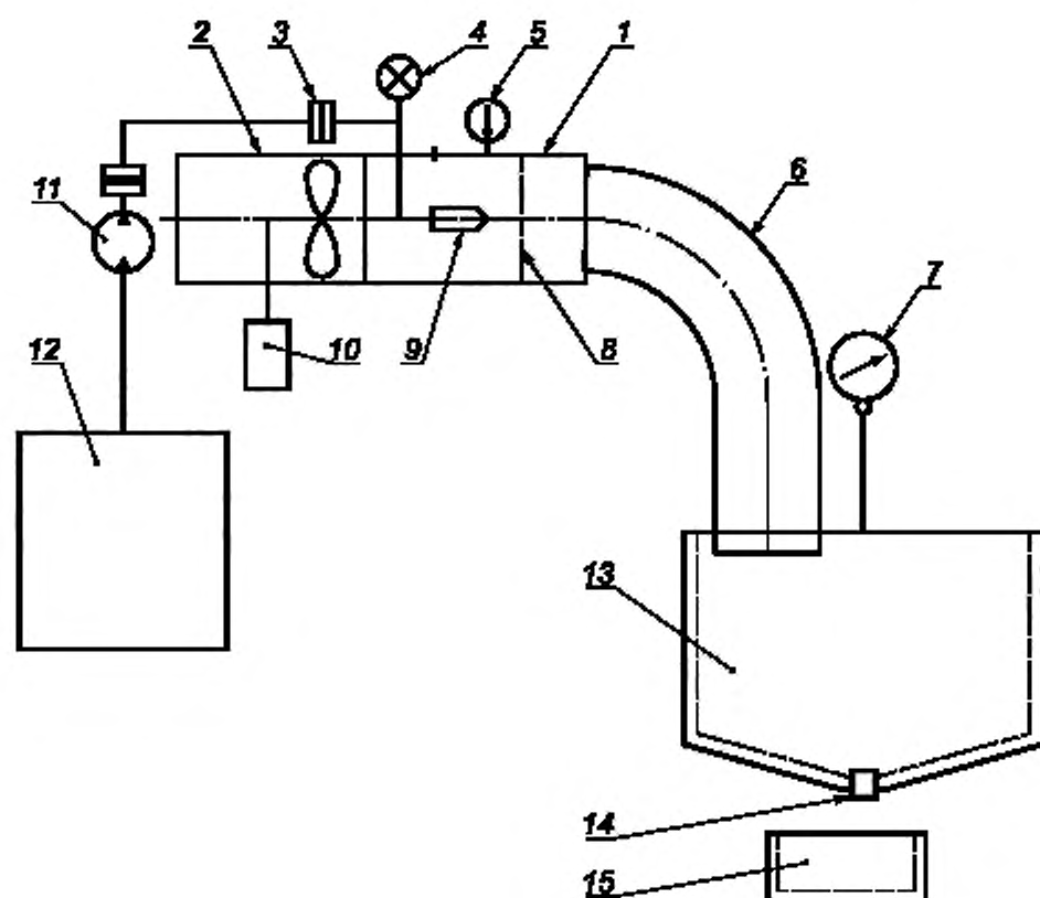
1 — ПГН; 2 — дымосос; 3 — соединение насосной установки с помощью пожарного рукава к распылителю ПГН; 4 — манометр; 5 — термометр; 6 — изгибательно-лентный рукав; 7 — подающие весы; 8 — сетка или перфорированная пластина; 9 — распылитель; 10 — привод дымососа; 11 — насосная установка; 12 — емкость с пенообразователем; 13 — емкость для сбора пены; 14 — пробка слива пенообразователя; 15 — емкость для сбора пенообразователя
