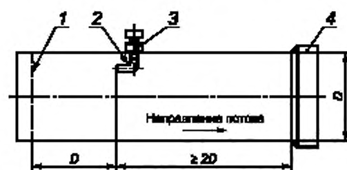
1 — выпрямитель струй потока; 2 — бобышка с приемником полного или комбинированного давления; 3 — датчик давления; 4 — присоединительный патрубок к корпусу дымососа
