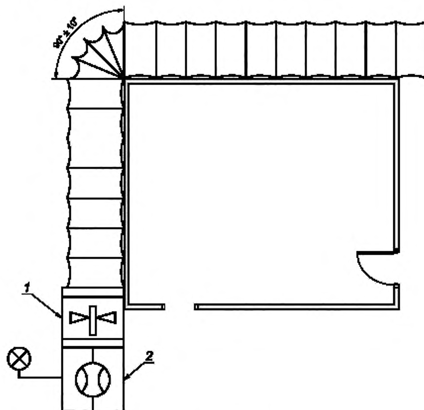
1 — дымосос; 2 — мерный воздухопровод
