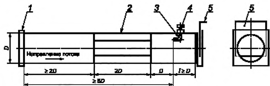
1 — присоединительный патрубок к корпусу дымососа; 2 — выпрямитель струй потока; 3 — бобышка с приемником полного или комбинированного давления по ГОСТ 12.3.018; 4 — датчик давления; 5 — дроселирующее устройство
