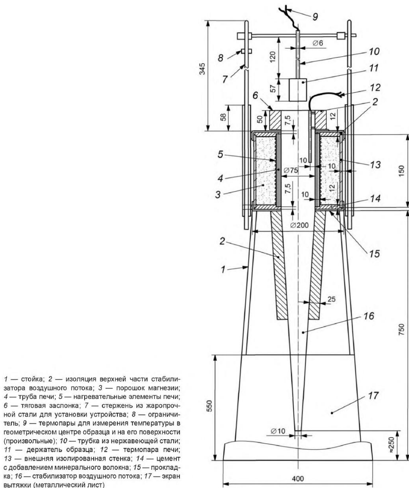
Рисунок А.1 — Типовое расположение оборудования установки для испытаний по методу I
