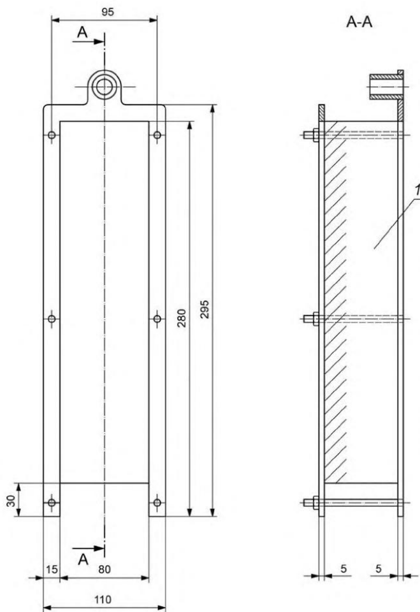
Рисунок Г.2 — Держатель образца для испытаний однослойных материалов
