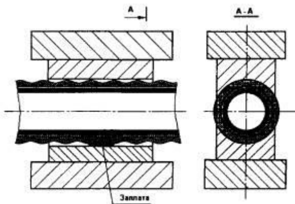
Рис. 6. Приспособление для ремонта посредством вулканизации
