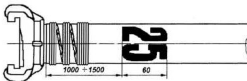
Рис. 4. Дополнительная маркировка рукава на рукавной базе
